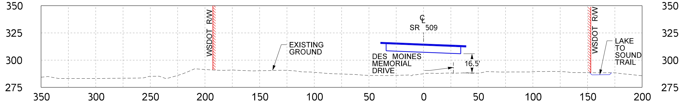
SECTION A-A
